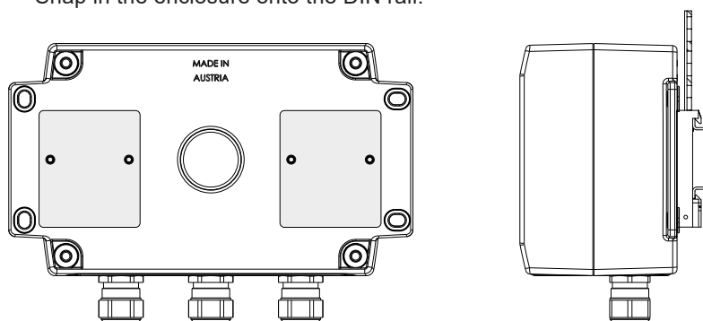
Fig. 27 DIN rail installation
